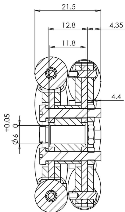
剖面 A-A
