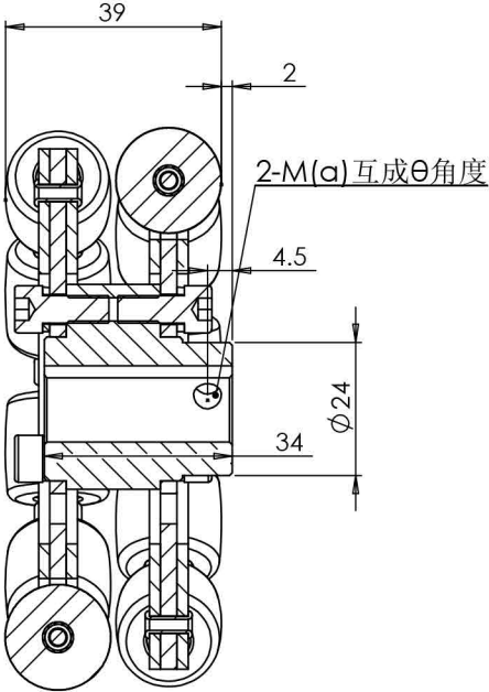
剖面 A-A
